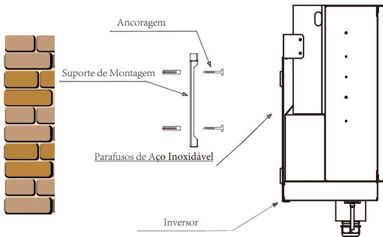
Figura 4.5 Instalação do Inversor
