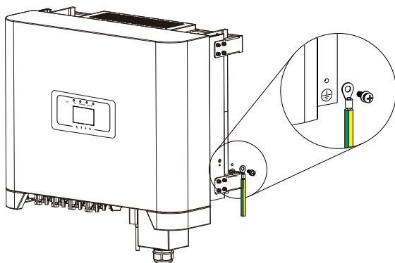
5.12 A Instalação do Aterramento da Carcaça
