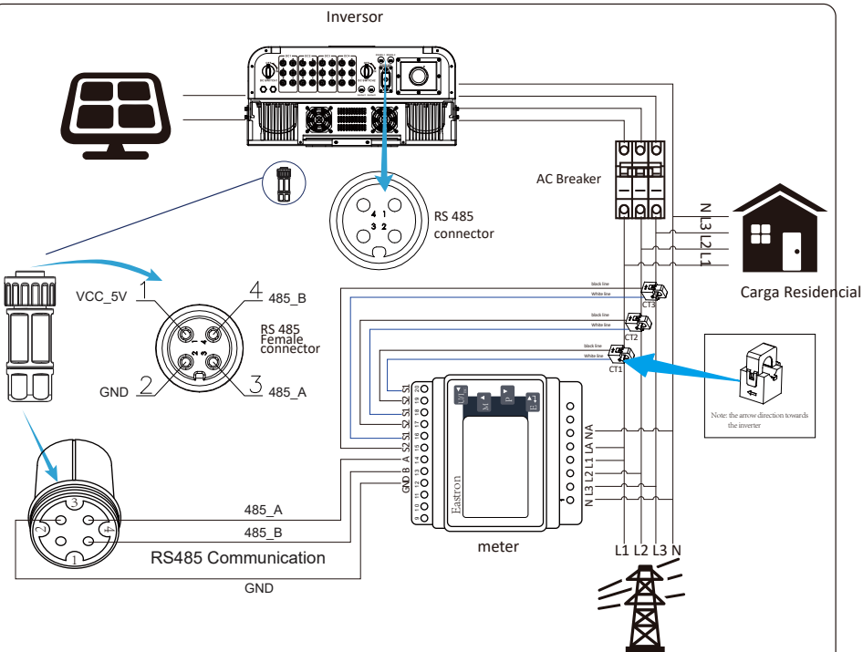
Figura 7.13 Diagrama de conexão com o medidor Eastron
