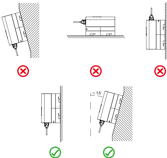
Figura 4.2 Ângulo de Instalação
