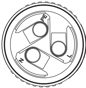
Figura 5.9 Padrão de furo do conector CA
