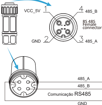
Figura 7.13 Diagrama da Comunicação do medidor Eastron
