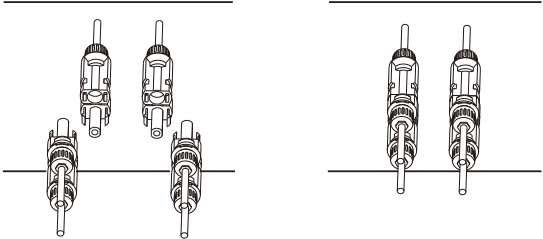
Figura 5.6 Conexão de Entrada CC
